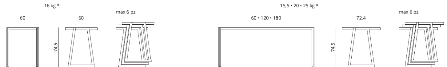
60 cm table / 120 cm table / 180 cm table
